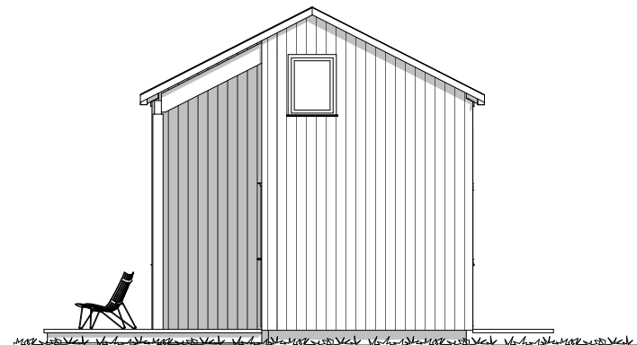
fasade D
