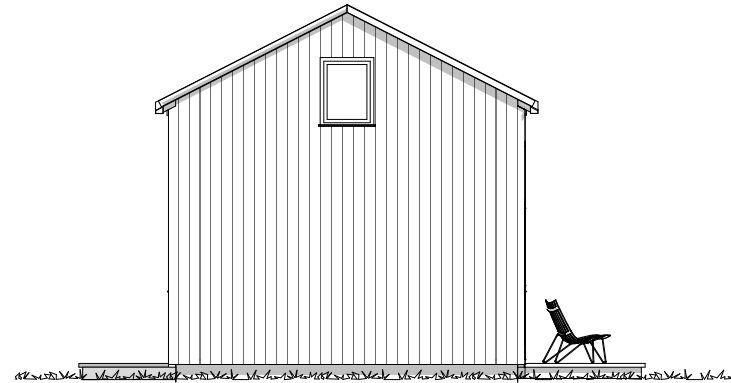
fasade B
